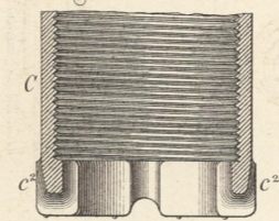
Fig. 12. M. 1:3.
