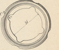
Bohrhütte Fig. 18. M. 1:100.
