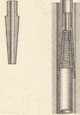
Fig. 10. M. 1:10. Fig. 11.
