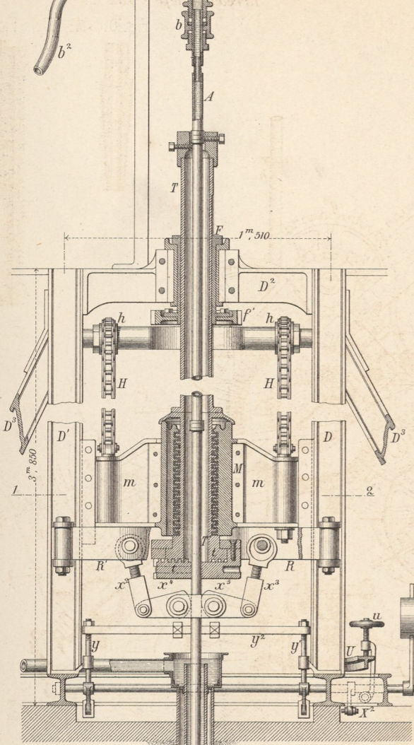
Fig. 2. M. 1:30.
