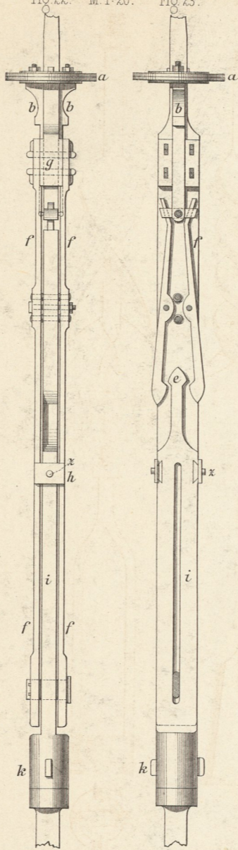
Nietamboß von Kind. Fig. 24. M. 1:36. Fig. 25.
