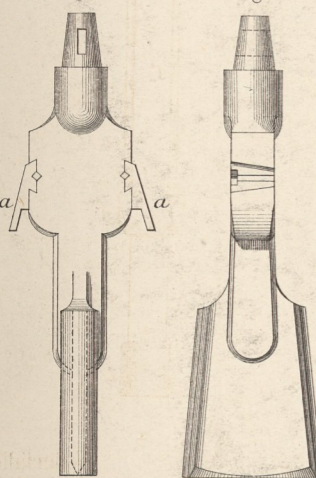
Laschenbohrer mit Nachscheiden. Fig. 8. M. 1:20. Fig. 9.
