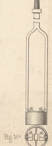
Klappenbüchse. Fig. 18 M. 1:36.
