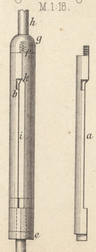
Freifallapparat von Fabian. Fig. 38. Fig. 39. M. 1:18.
