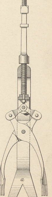
Eisenfänger. Fig. 41 M. 1:15.
