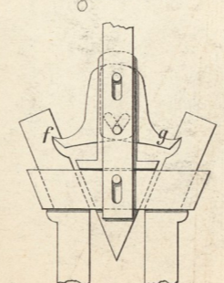
Eicken'sche Arretirung Fig. 26 M. 1:2.
