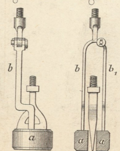
Nietamboß von Kind. Fig. 24. M. 1:36. Fig. 25.
