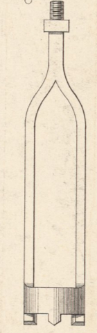
Kind'sche Bohrbüchse. Fig. 10. M. 1:30.
