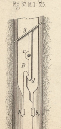
Freifallapparat von Greiffenhagen. Fig. 37 M. 1:25.
