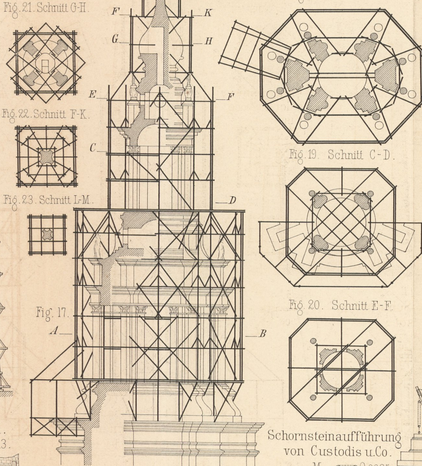
Gerüst für die Turmspitze der Cathedrale zu Chalon.
