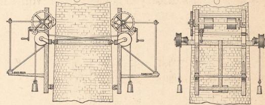
Maschine zum Besteigen von Säulen und Kaminen.
