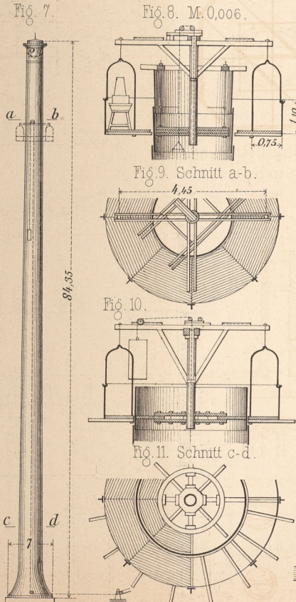
Fig. 7 bis 11. Schmiedeiserner Schornstein in Creusot.
