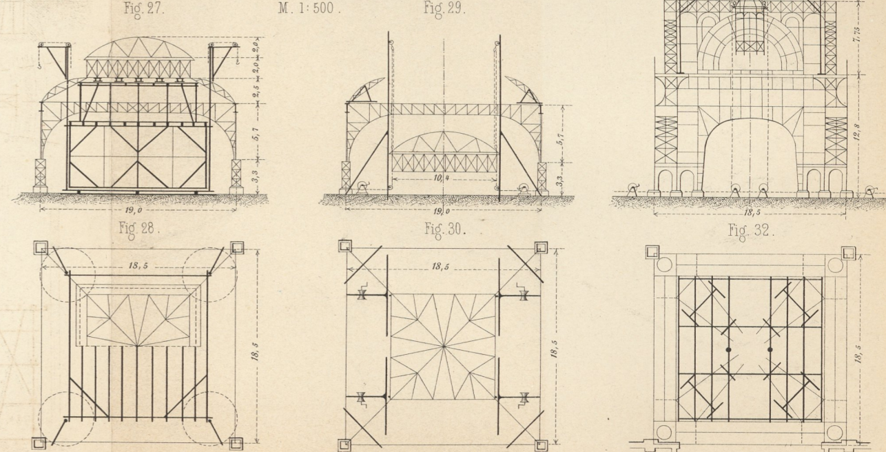
Aufstellung des Hauptgebäudes der Hygiene-Ausstellung in Berlin 1883.
