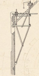
Hebe gerüst (zu Fig. 1.)
