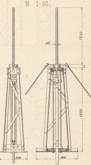
Hebevorrichtung.
