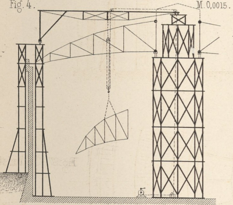
Projekt der Montirung eines Gasometerdaches ohne Zugring.
