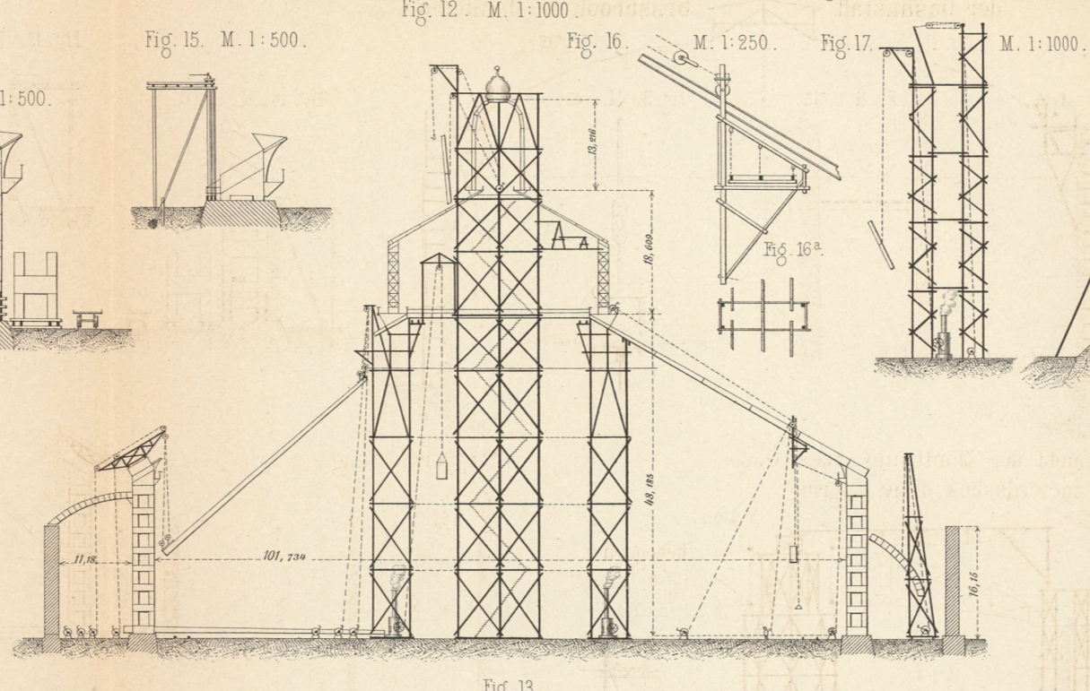
Rotunde der internationalen Ausstellung Wien 1873. (Fig. 12-22.)
