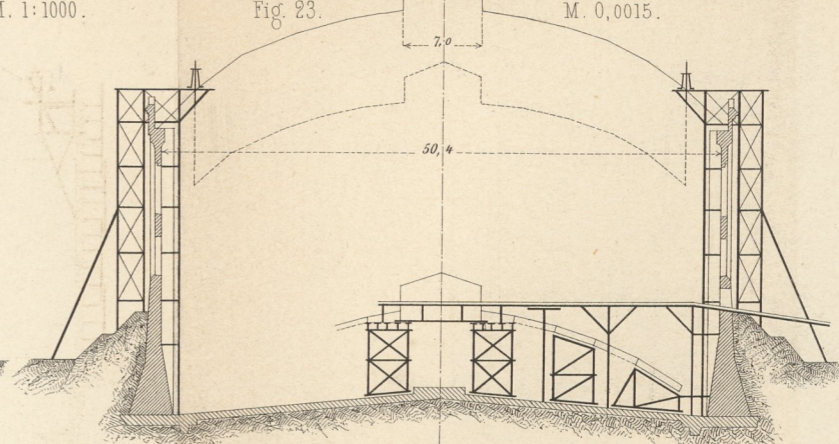
Mauergerüst, Montirungs- und Hebe gerüst für den Teleskopgasometer der III Dresdener Gasanstalt.
