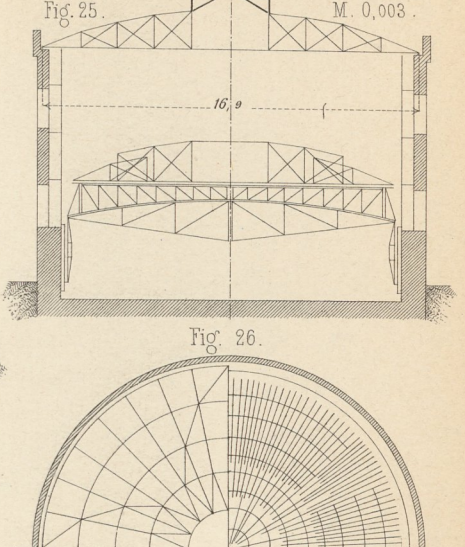
Montirung des Gasometerdaches in Berlin Hellweg 8.
