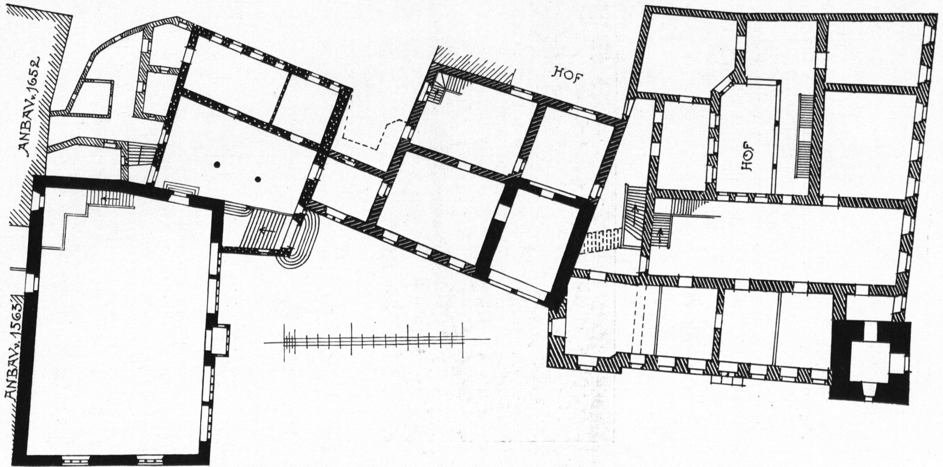
Abb. 160. Rathaus zu Regensburg. Grundriß des ersten Stockwerks. Nach einer Aufnahme des Stadtbauamts.
