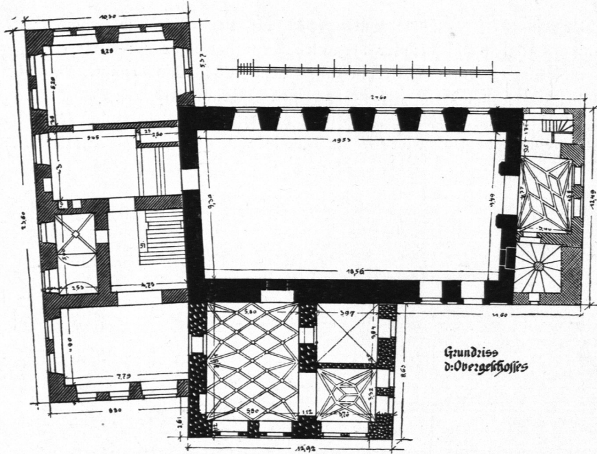
Abb. 148. Rathhaus zu Gardelegen. Grundriß des ersten Stockwerks.
