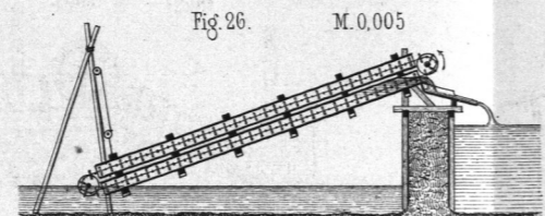
Geneigtes Schaufelwerk. M. 0.005.
