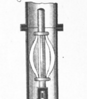
Doppelt wirk Pumpe. Fig. 50. M. 0.030.
