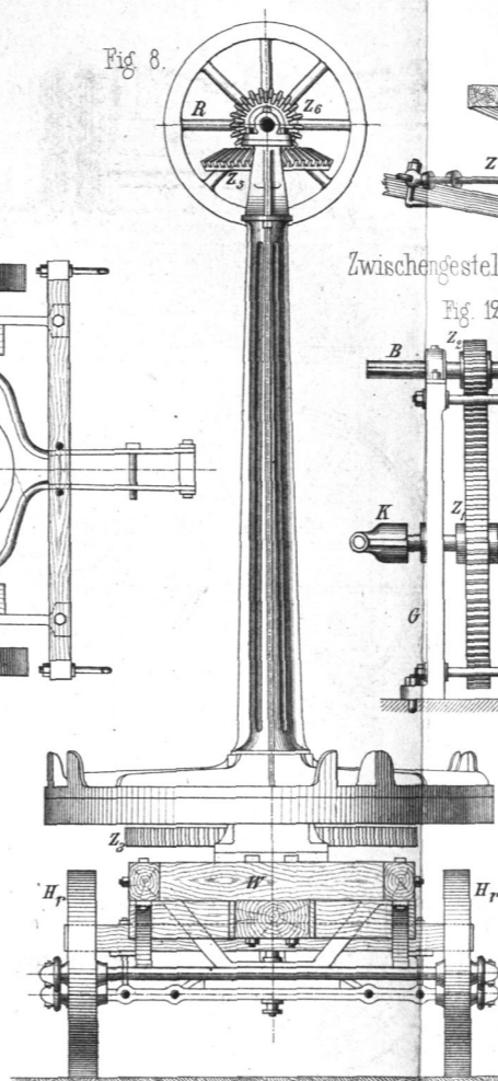
Vierpferdiger fahrbarer Säulengöpel von H. Lanz in Mannheim. M. 0,04.
