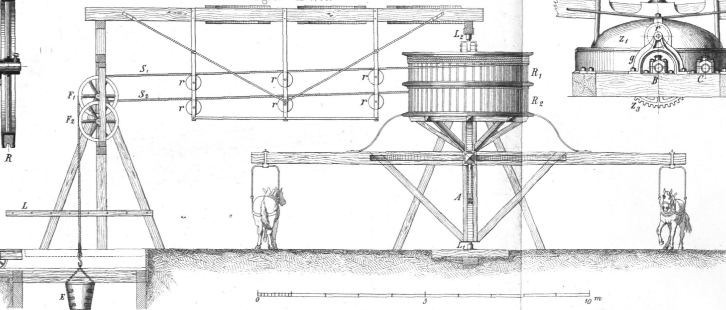
Pferdegöpel für Schachtförderung. Fig. 18. M. 0,009.
