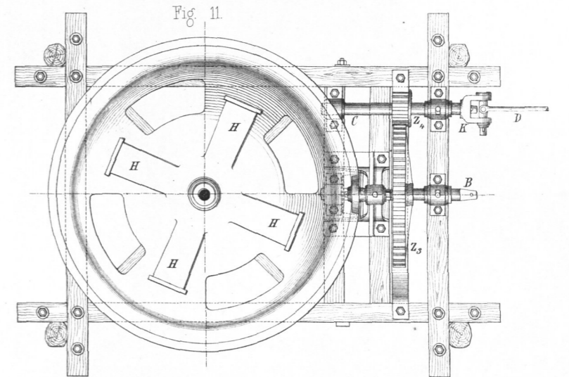
Bergner's zweipferdiger Glockengöpel.
