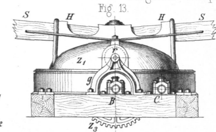
Bergner's zweipferdiger Glockengöpel.
