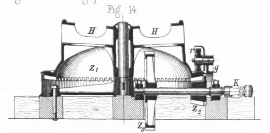
Bergner's zweipferdiger Glockengöpel.
