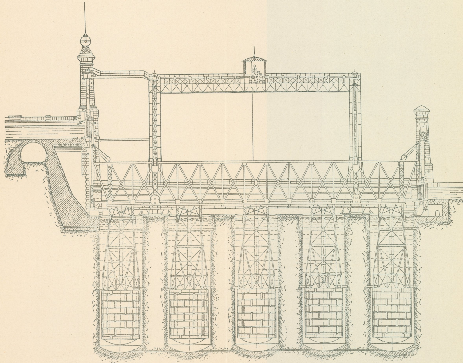
Längsschnitt
