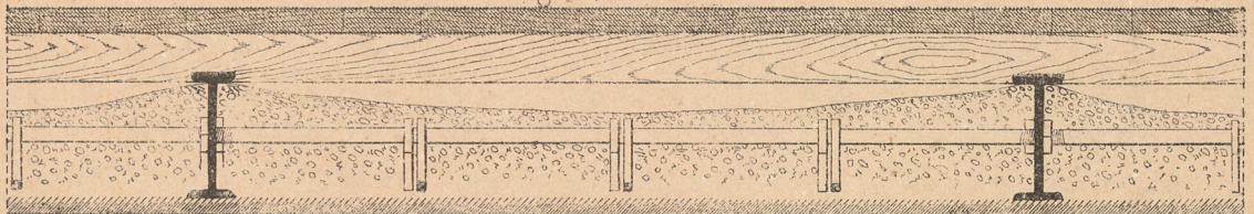
Fig. 4. Schnitt C' D'.
