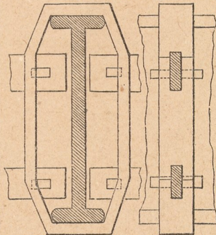
Detail IX. Fig. 6.
