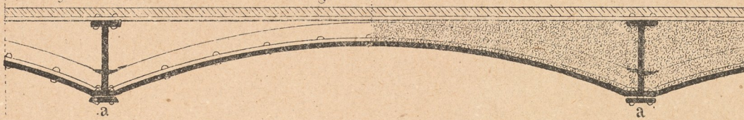
Fig. 2. Schnitt CD.
