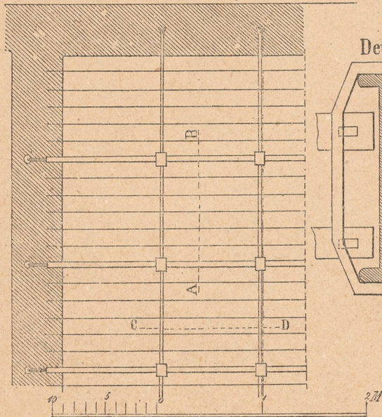
Grundriss zu IX u. X. Fig. 5.
