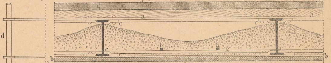
Fig. 4. Schnitt G H.
