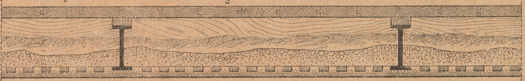
Fig. 4. Schnitt C'D'.
