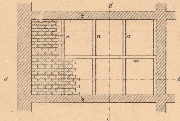
Fig. 2. Grundriß des ersten Stocks.
