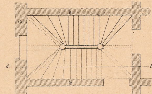
Fig. 2. Grundriß des ersten Stocks.
