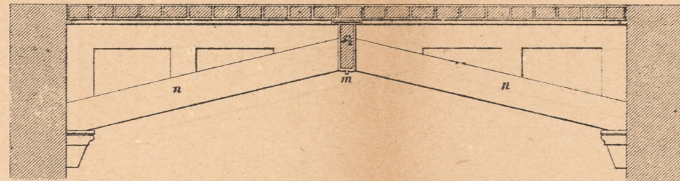
Fig. 6. Längendurchschnitt der Decke nach a b.
