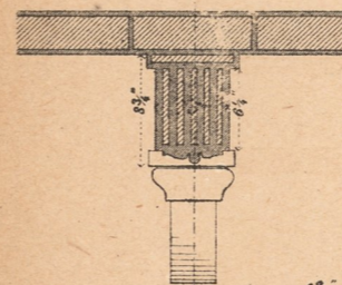
Fig. 9. Durchschnitt der Stufen nach n o.
