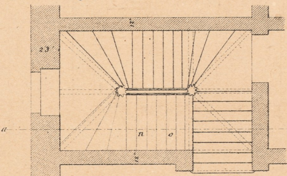
Fig. 1. Grundriß des Erdgeschosses.
