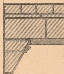
Fig. 7. Längendurchschnitt eines Trägers unter dem Podeste.
