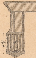
Fig. 10. Durchschnitt der Treppenwange nach e f g.
