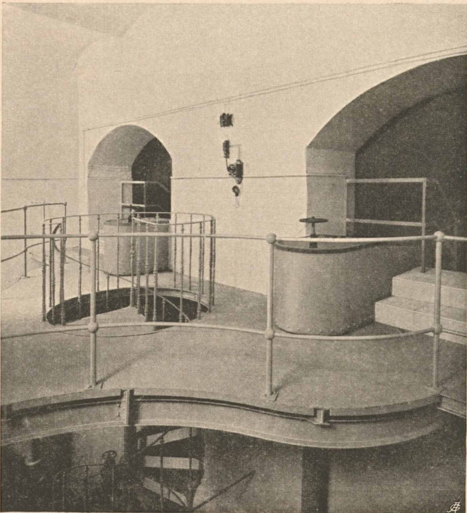
Nr. 168. Höchstreservoir Kobenzl (Innenansicht der Schieber- kammer).
