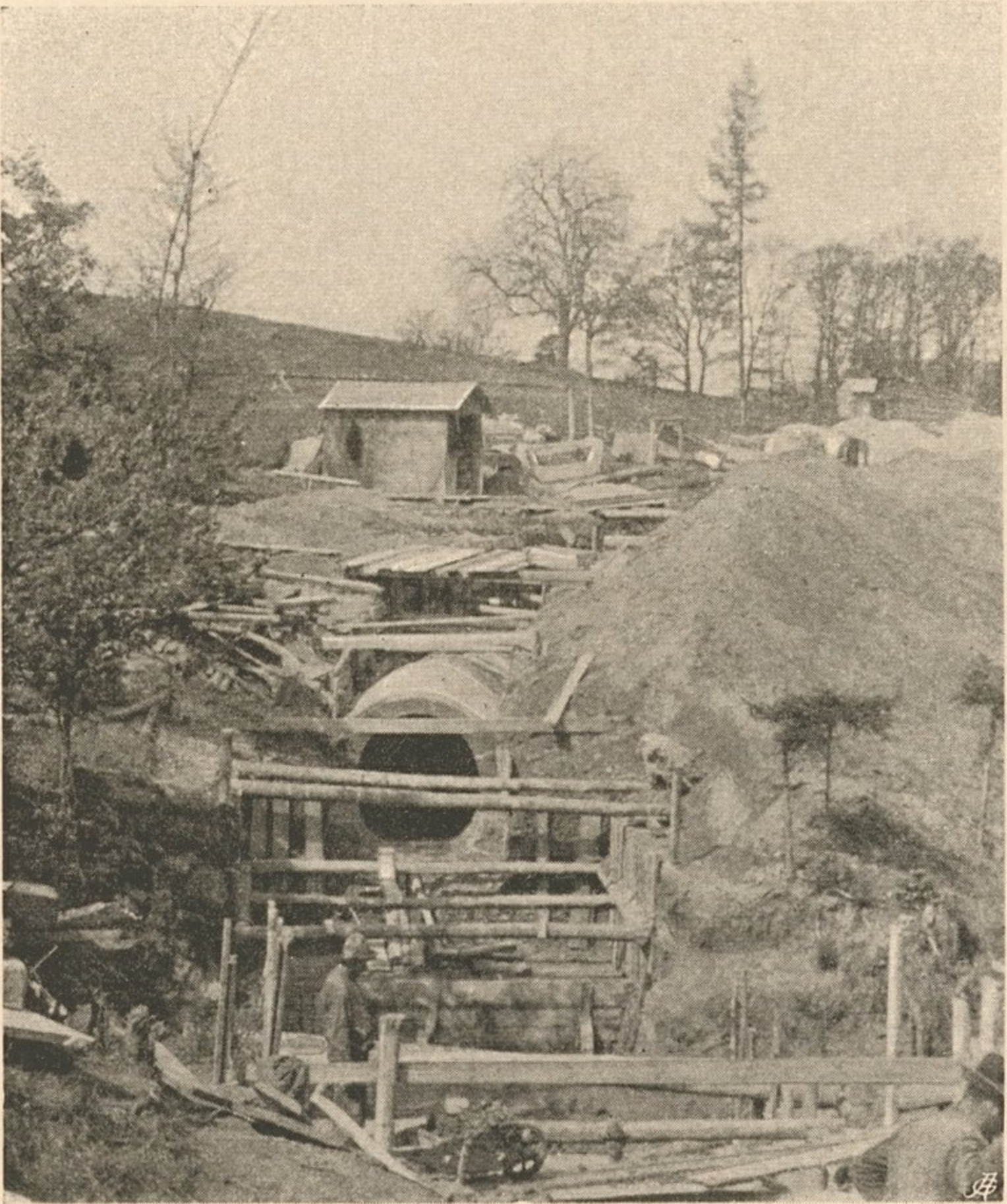
Nr. 116. Bau des Leitungskanales bei Fabrafeld.
