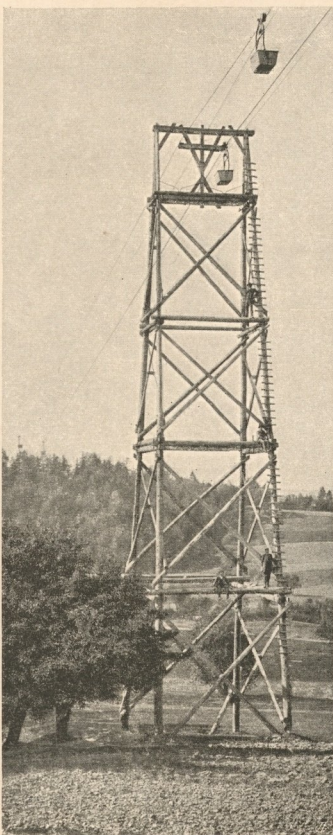
Nr. 79. Ständer einer Drahtseilhänge- bahn im Tale der Melk.
