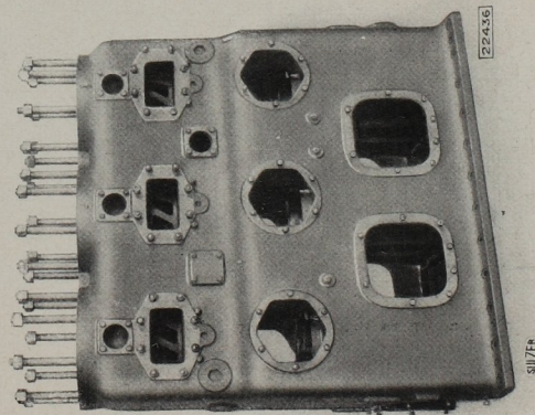
Blockeinheit mit 3 Zylindern
