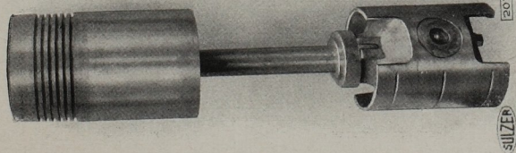
Kolben mit Kreuzkopf
