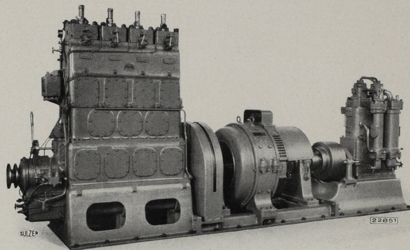
100 PS. Vierzylinder-Sulzer-Zweitaktschiffsdieselmotor mit luftloser Einspritzung, direkt gekuppelt mit Dynamo und Kompressor
