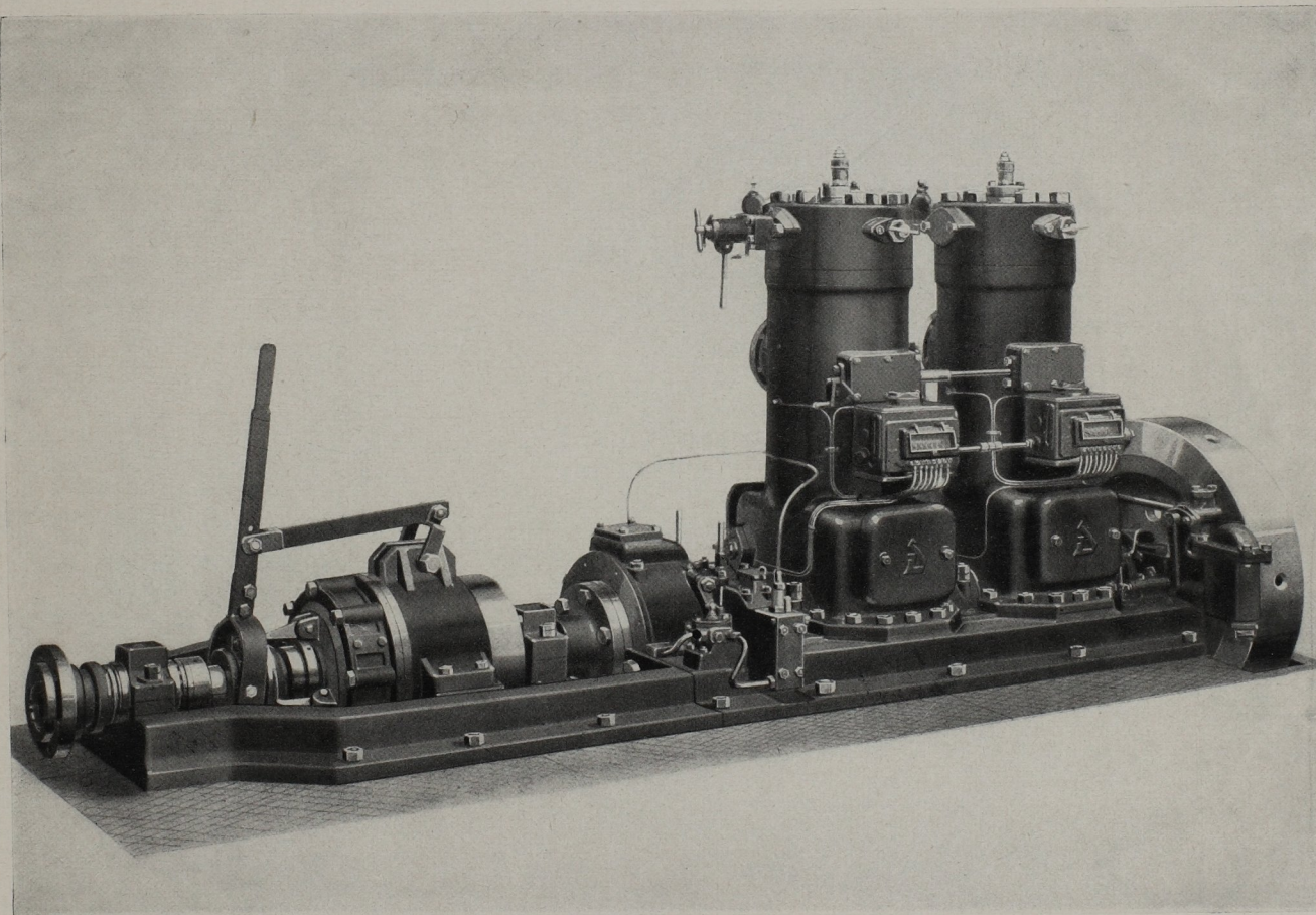
Kompressorlose Zweitakt-Dieselmachine für Bootsbetrieb Bauart 2 KZ 32 mit Wendegetriebe, Leistung 70 PS e , n = 375 , Gewicht netto 5540 kg
