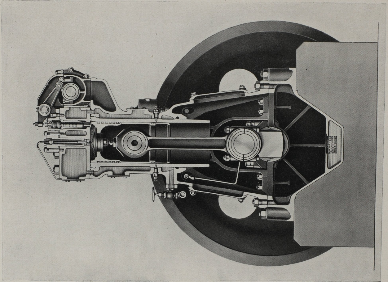
Querschnitt durch einen kompressorlosen Dieselmotor, Type KS 20, mit N = 15 \div 25 PS bei n = 300 \div 500 . Ausführung in 2-6 Zylindern
