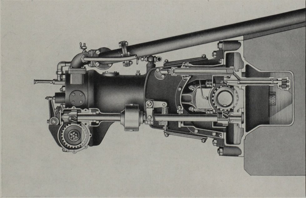
Schnitt durch Steuerwellen- und Schmierpumpenantrieb eines kompressorlosen Dieselmotors, Type KS 20
