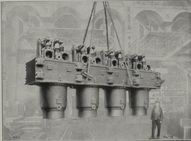
Zylinderblock im Kran hängend
