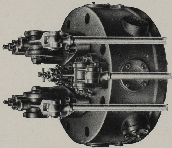
Zylinderkopf eines kompressorlosen Standard-Dieselmotors
