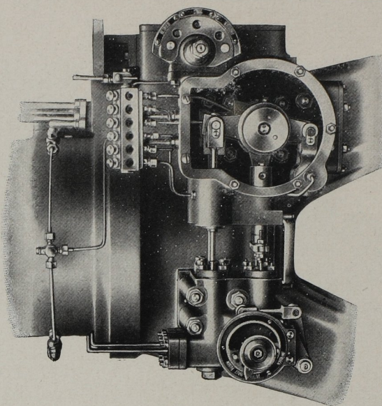
Brennstoffpumpe eines Dieselm. mit Kompressor
