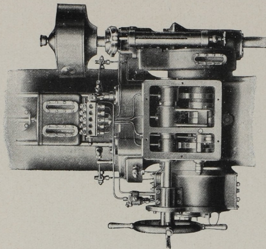
Steuerwelle und Triebwerkkasten eines Dieselmotors mit Kompressor
