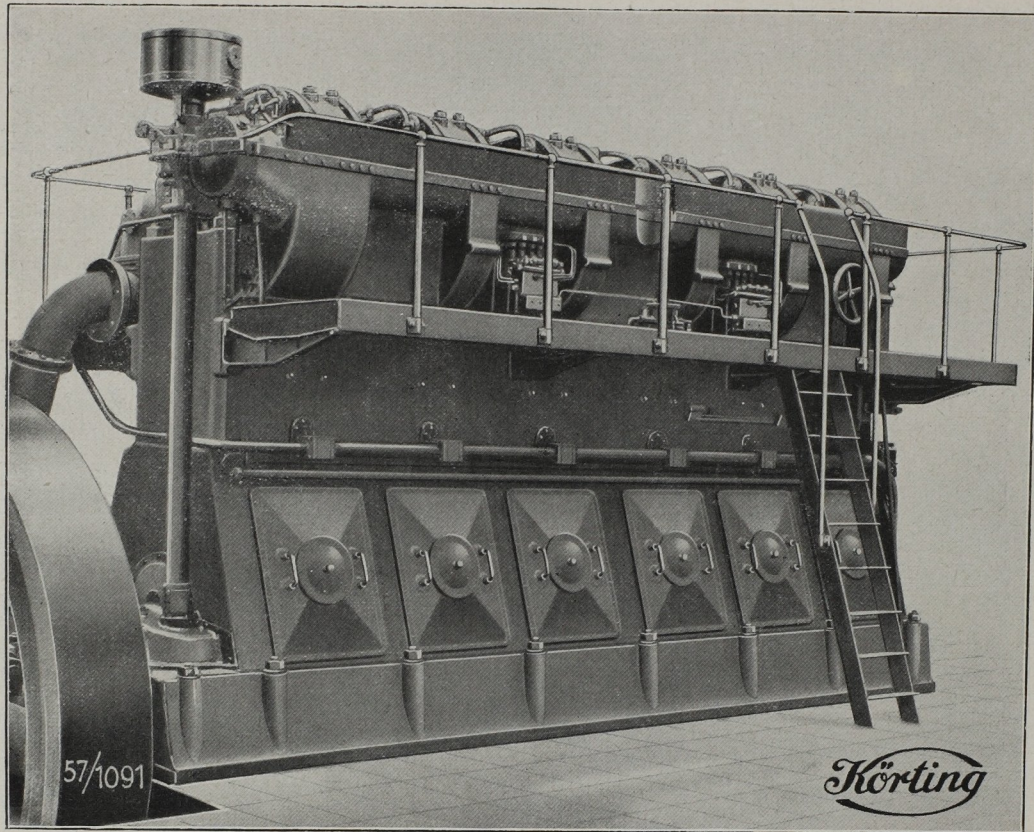
1200 PS stehende Körting-Dieselmachine ohne Kompressor
