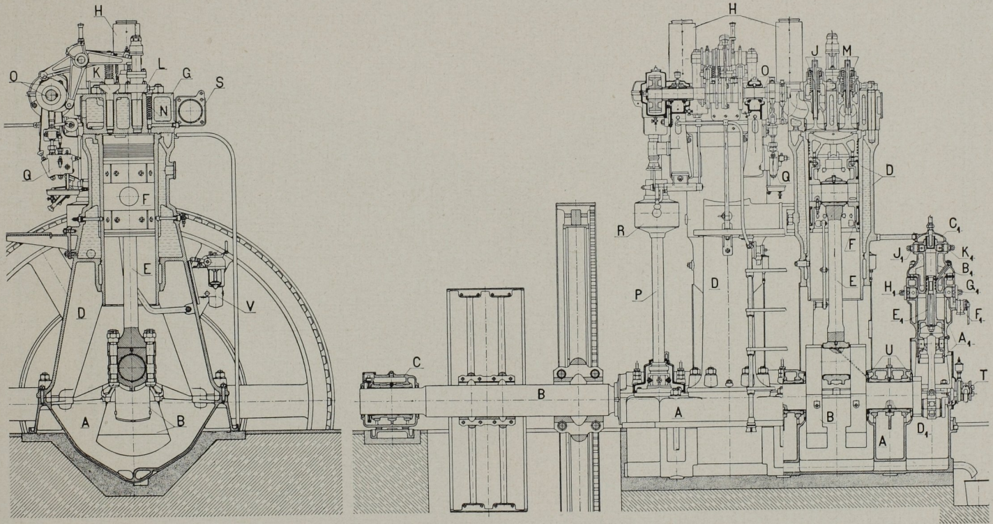
Schnitt durch eine Zweizylinder-Viertakt-Dieselmachine (NS-Motor)
