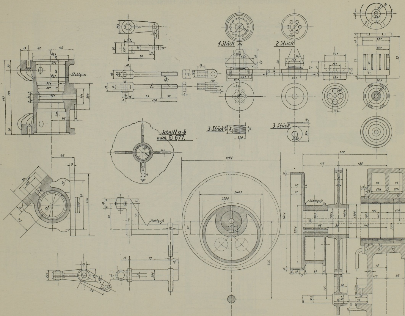
Ventile mit Gehäuse, Exzenter für die Wasserpumpe und Kupplungshälfte für Kupplung nach ⌀ 681.
