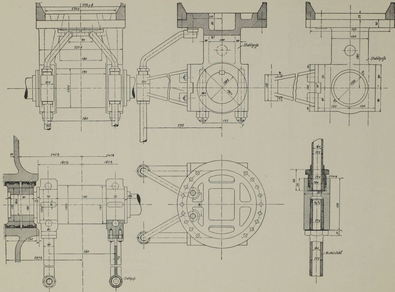
Kreuzkopf (unterer Teil des Kolbens) mit Posaunenrohren für Kolbenkühlung.
