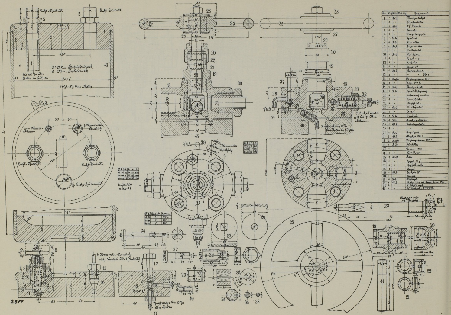
Beschreibung unter D 110 in Band I. Schaltung der Rohrleitungen nach D 111a; Wahl der Leitungen nach D 111b; Verschraubungen nach D 114 und D 317a.
