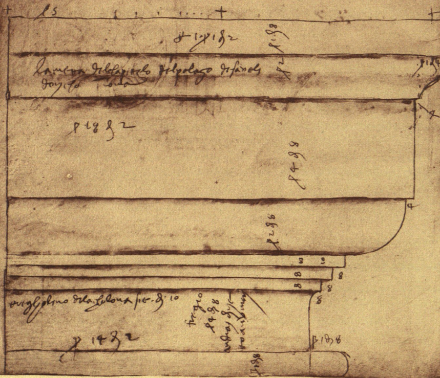
CHAPITELO DORICO A SANTO PIERO I. GRADO APISA
