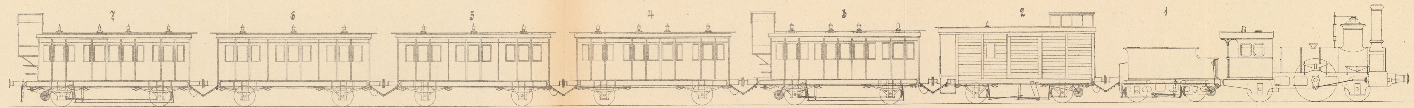
1... Tender mit Bremse und Hebovorrichtung 2, 3, 7... Bremswagen 4, 5, 6... Zwischenwagen mit Leitung
