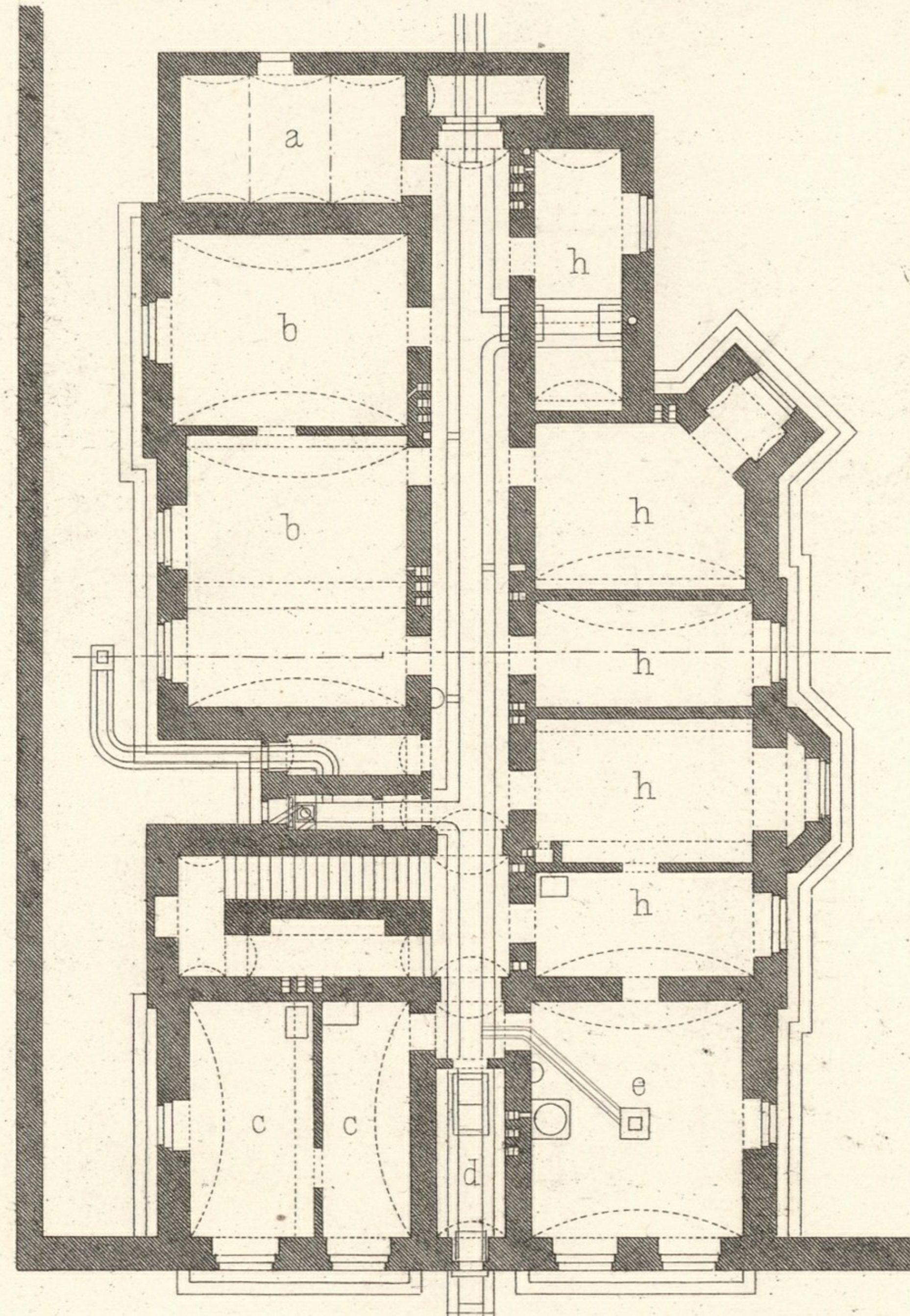
SOUTERRAIN. — SOUS-SOL.
