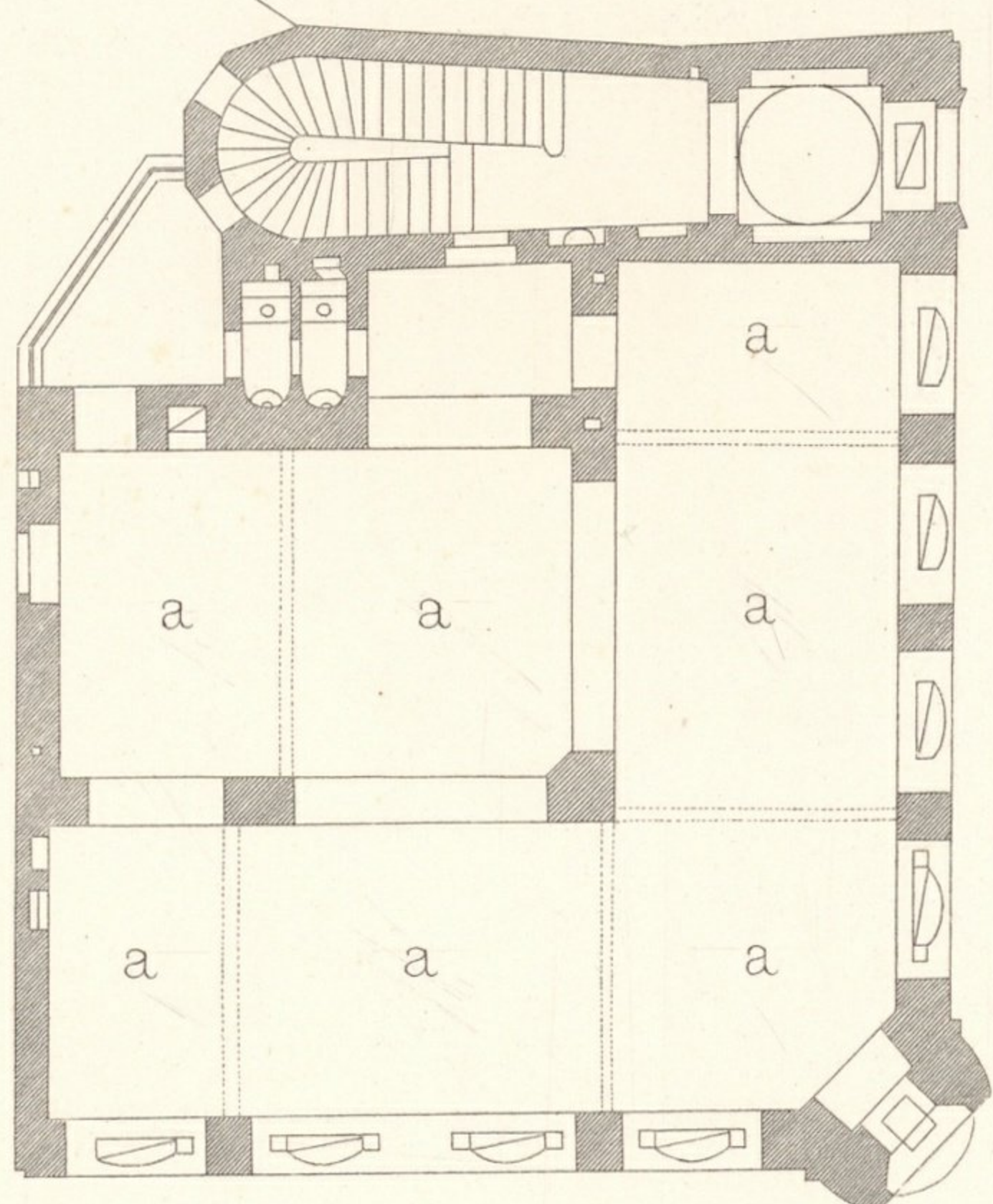
ERDGESCHOSS. — REZ-DE-CHAUSSÉE.
