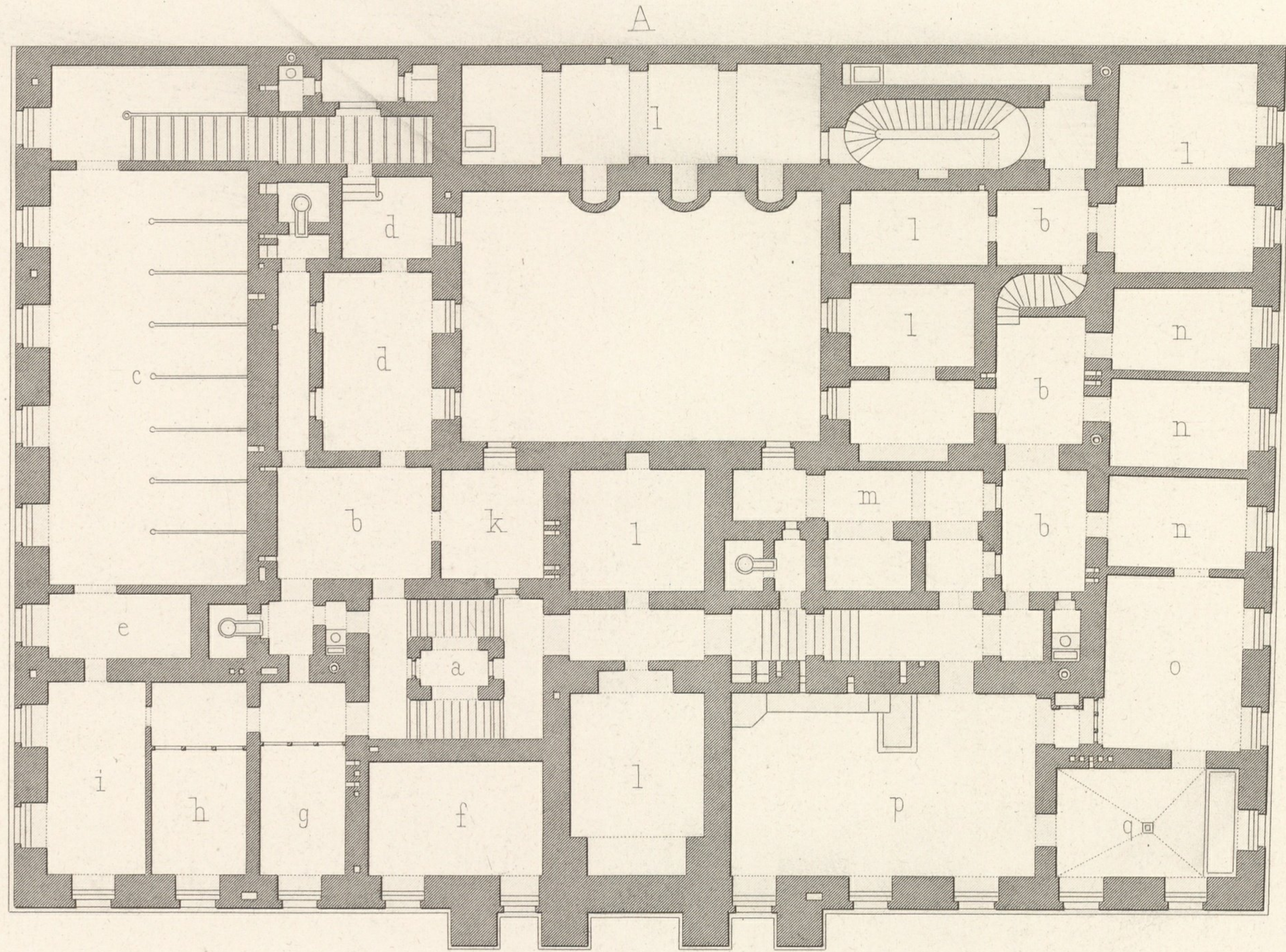
A. UNTERGESCHOSS.
