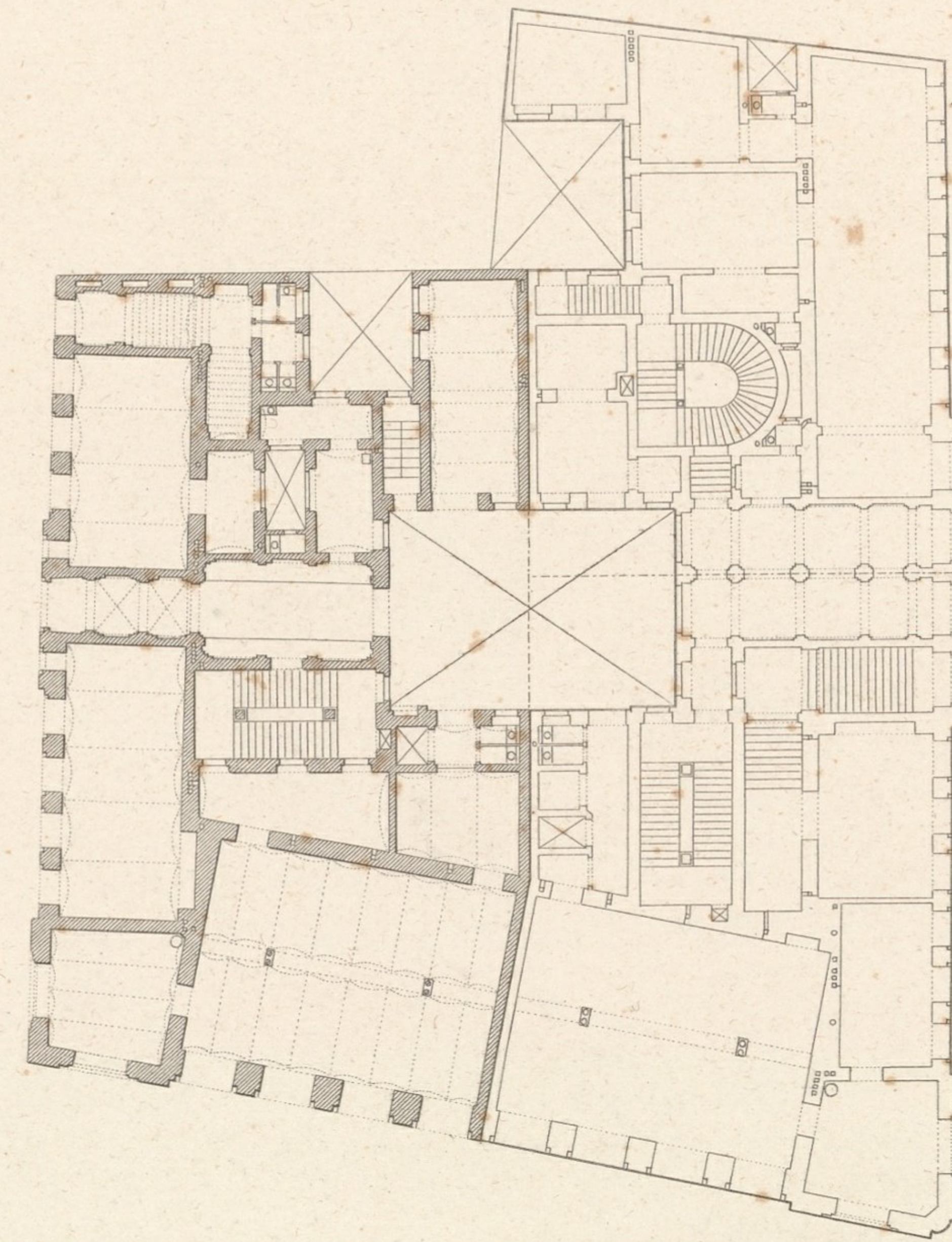
A. ERDGESCHOSS. B. STOCKWERKE. A. REZ DE CHAUSÉE. B. ETAGES.
