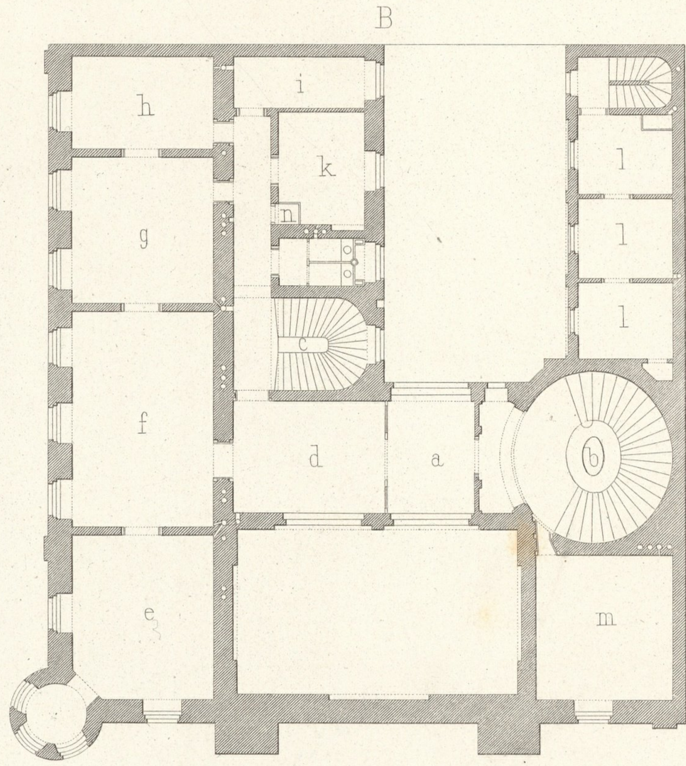
B. ZWISCHENGESCHOSS
