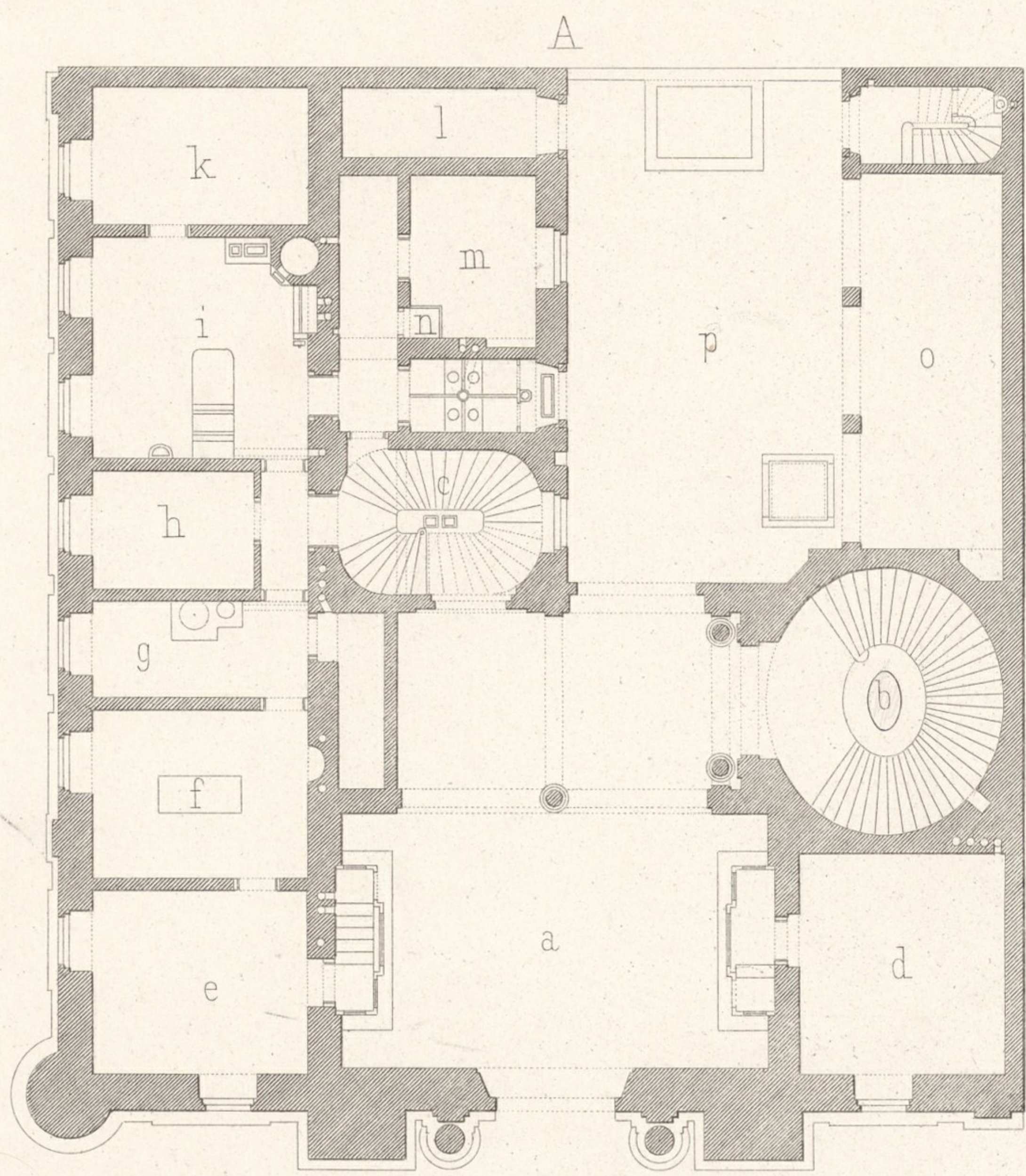
A. ERDGESCHOSS
