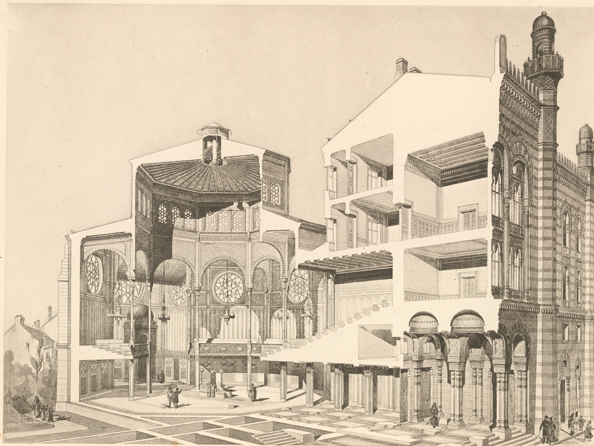
Neue Synagoge in Buda-Pest perspectivischer Schnitt.
