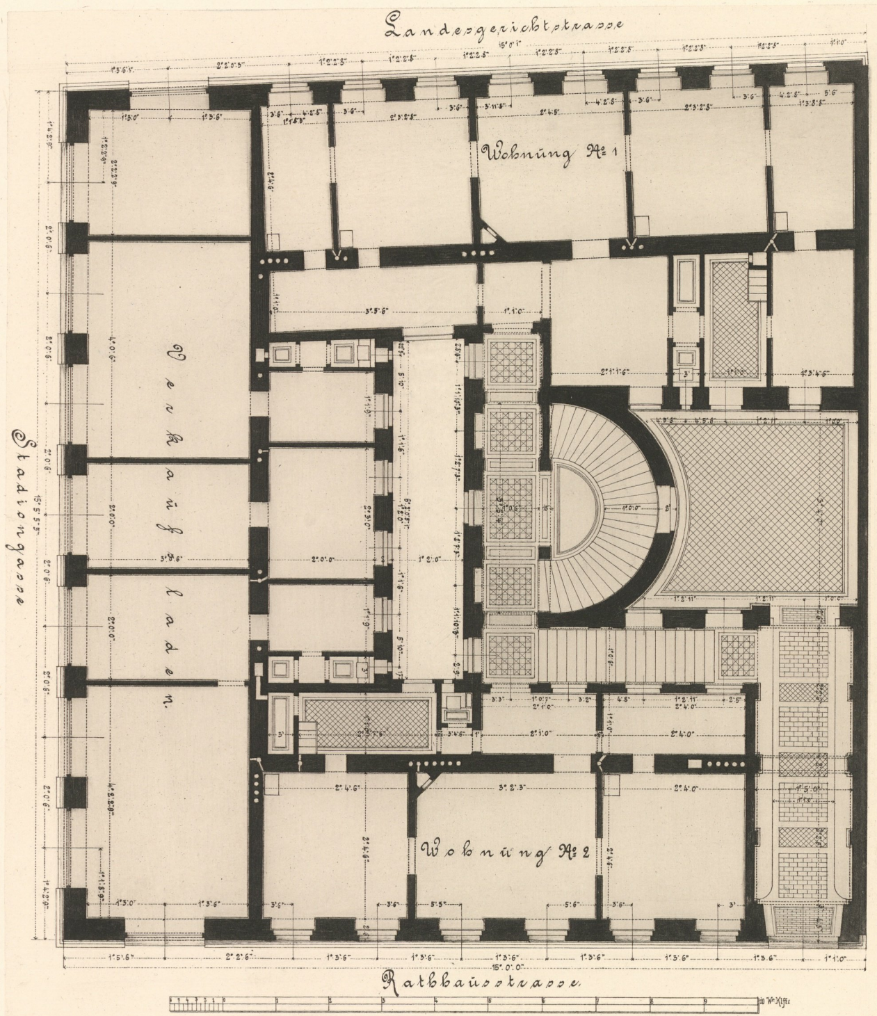
Miethaus I. Rathaus-Strasse 3 Grundriss des Parterres.
