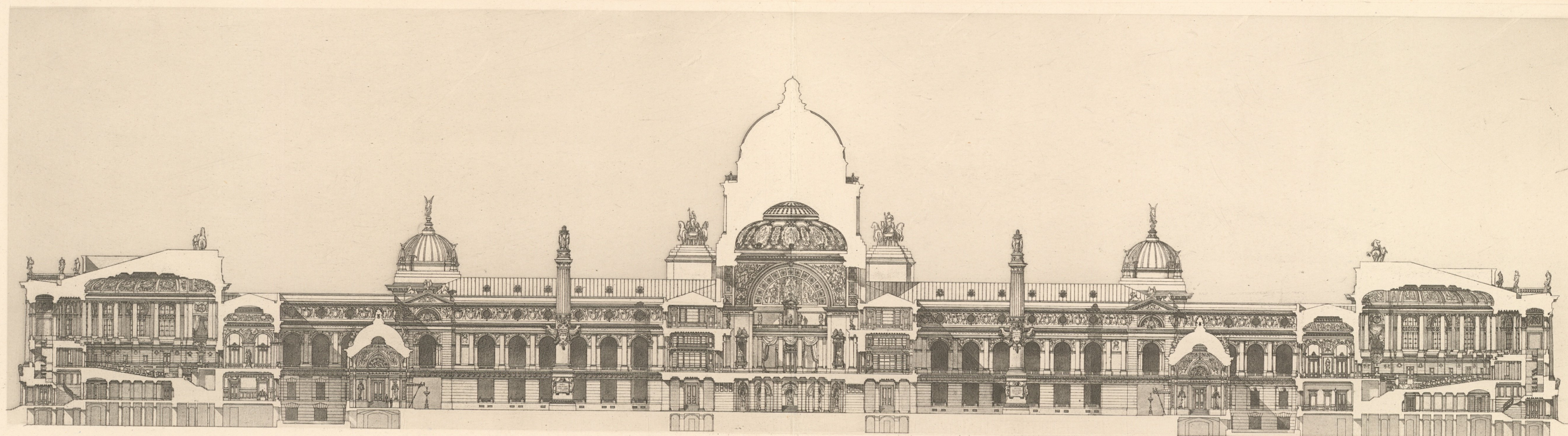
Parlaments-Gebäude in Buda-Pest Concursproject. - Längenschnitt.
