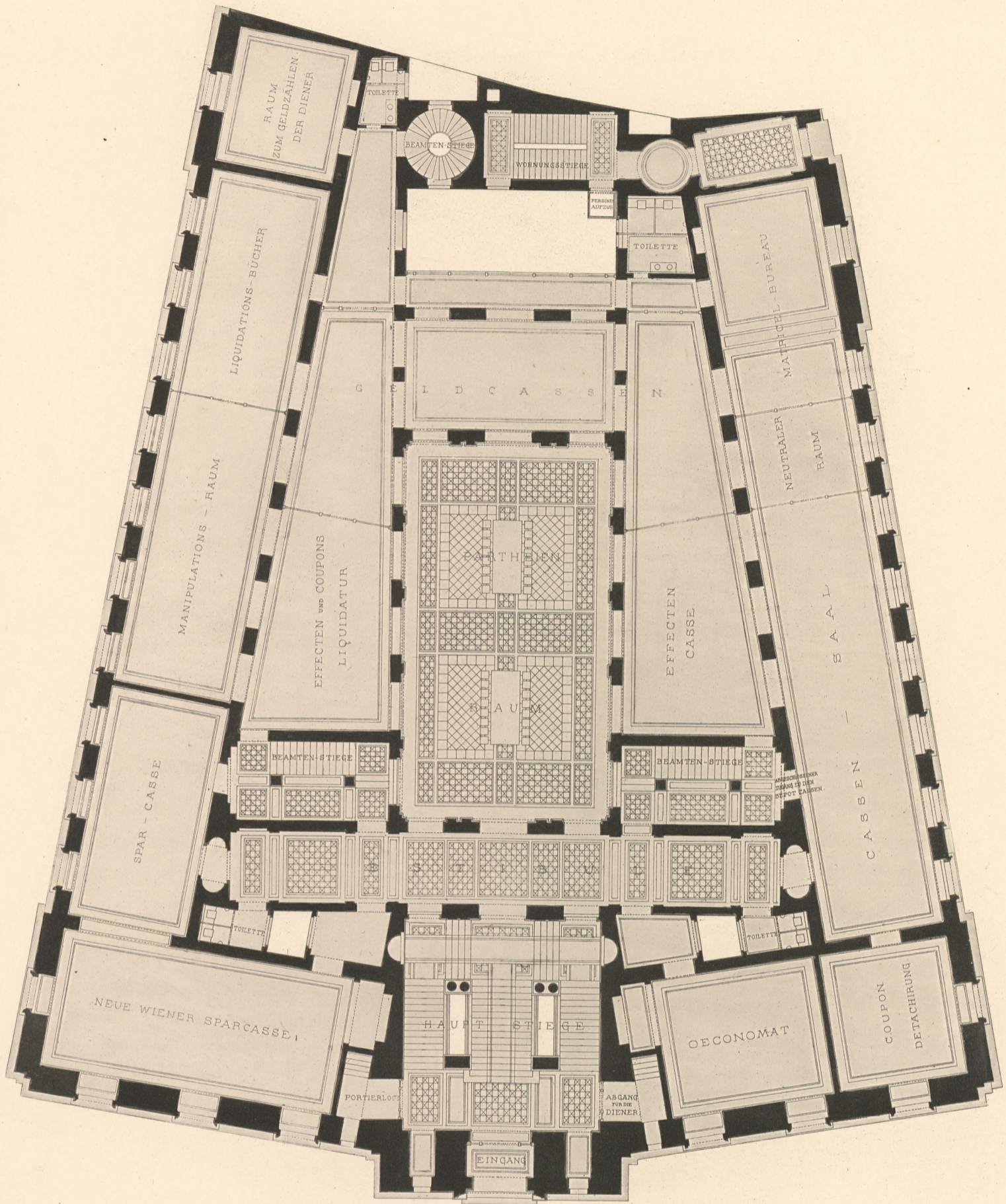
Amtsgebäude der k.k. priv. allgem. österreichischen Boden-Creditanstalt Concurproject - Grundriß des Parterres.
