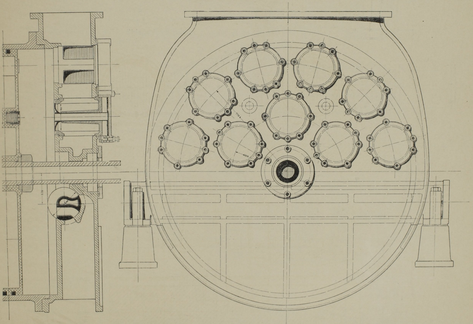
Abb. 86. Querschnitt durch den Windcylinder und Längsschnitt durch den Deckel. Masst. 1 : 15.
