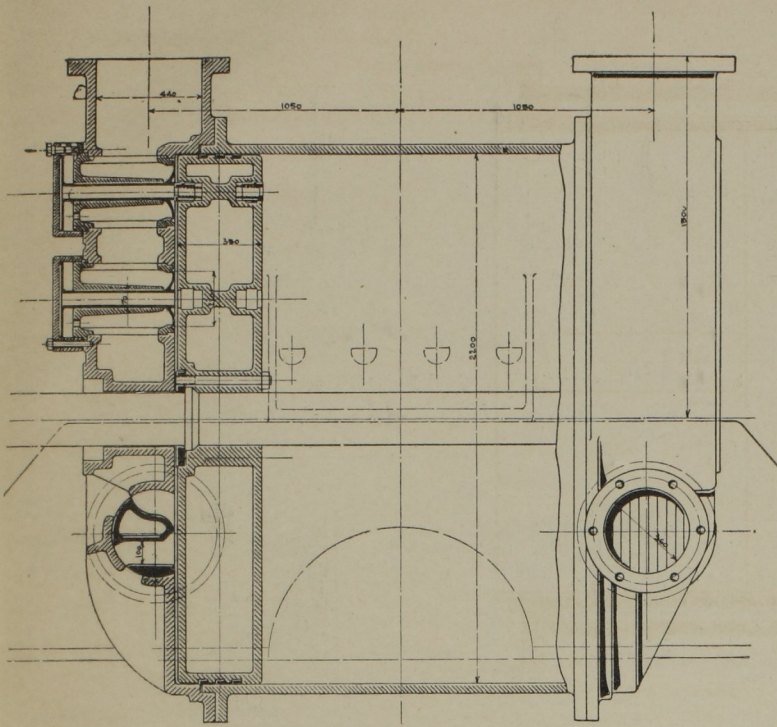
Abb. 84. Längsschnitt des Windcylinders. Masst. 1 : 30.
