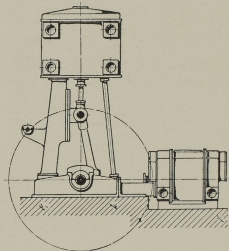
Abb. 50 a. Seitenansicht.
