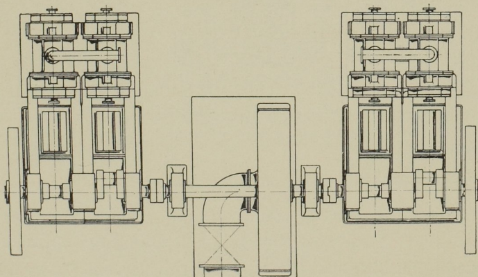
Abb. 47a. Grundriss.
