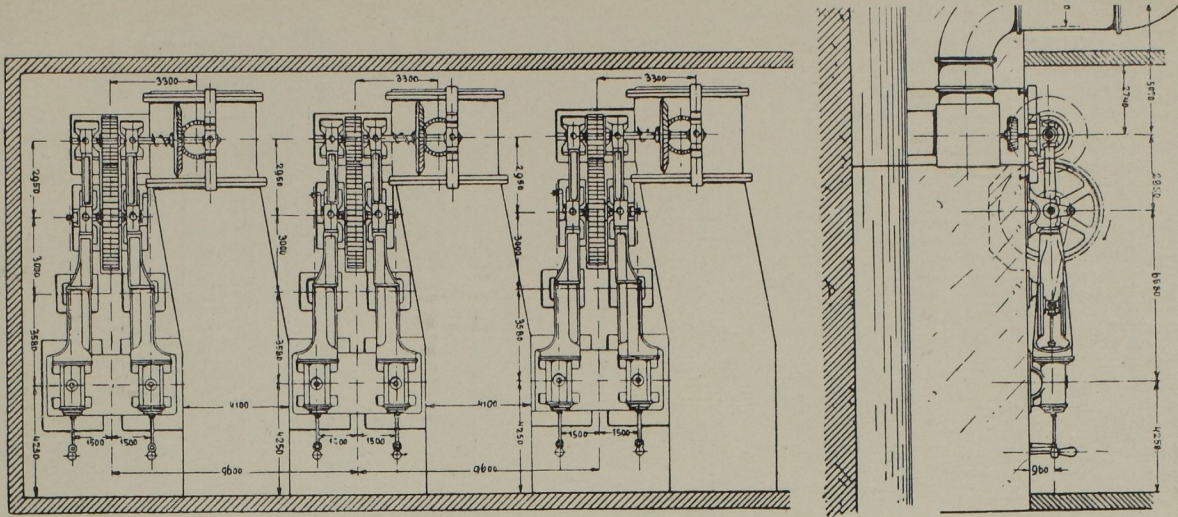
Abb. 39. Kompressor-Anlage der Chapin-Mine in Iron Mountains, Michigan. Masst. 1:275.
