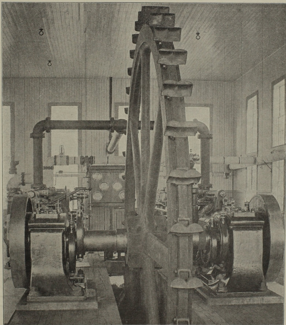
Abb. 82. Peltonrad-Antrieb.
