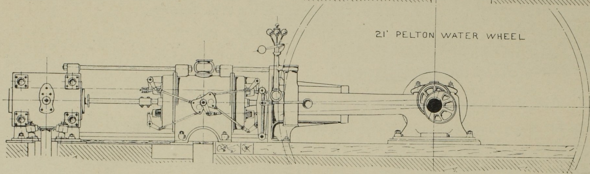
Abb. 79. Seitenansicht. Masst. 1:72.
