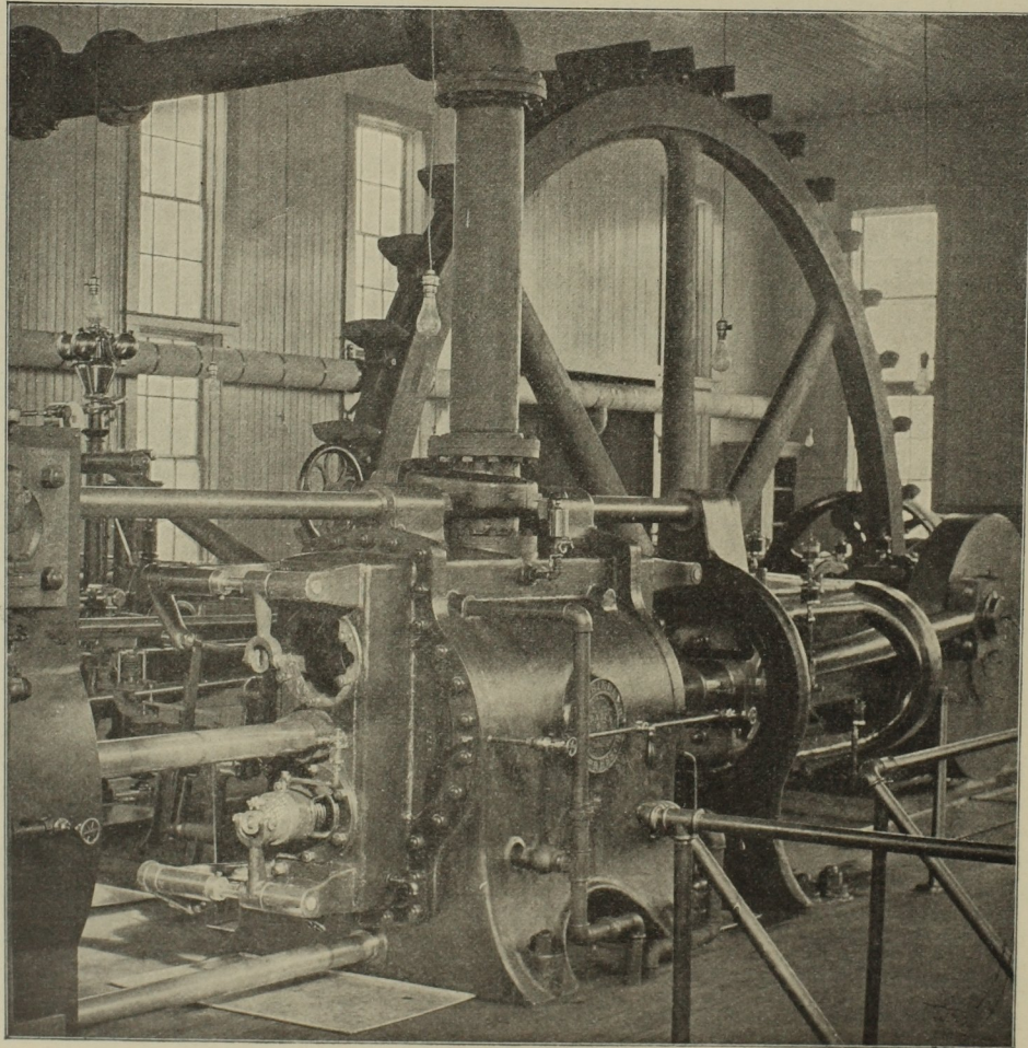
Abb. 80. Gesamtbild des Kompressors mit Antrieb. Verbund-Kompressor für die Alaska Treadwell Gold Mining Co., gebaut von Fraser & Chalmers in Chicago.
