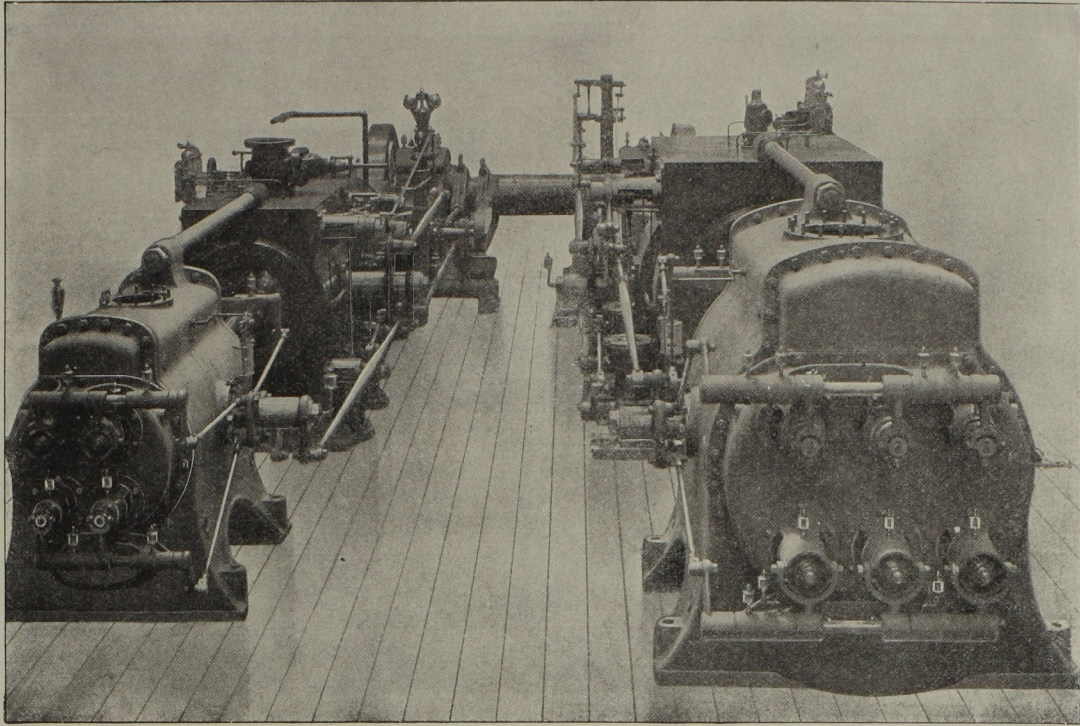
Abb. 75. Gesamtansicht des Kompressors und seiner Steuerung.
