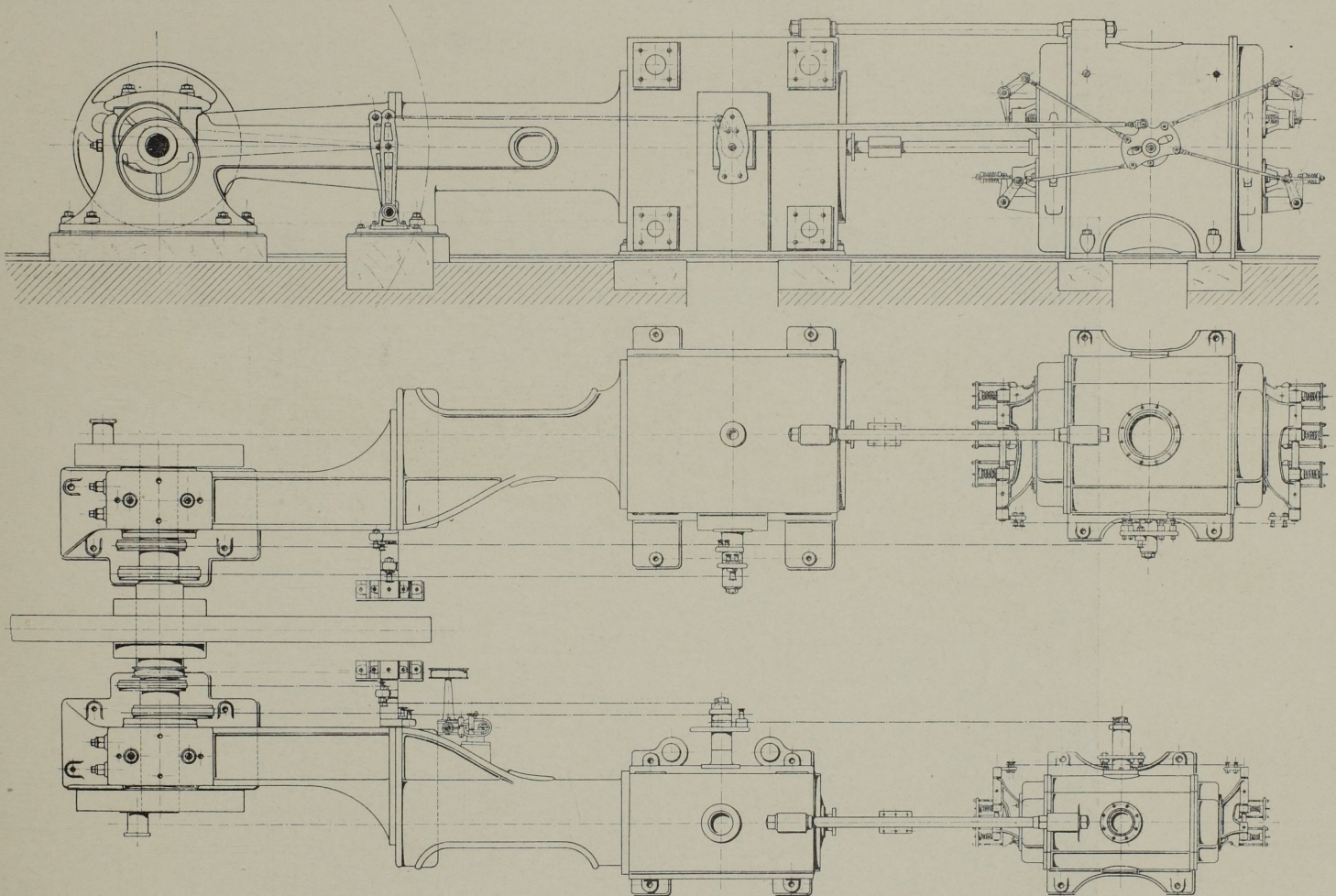
Abb. 76. Grundriss. Massst. 1 : 64.
