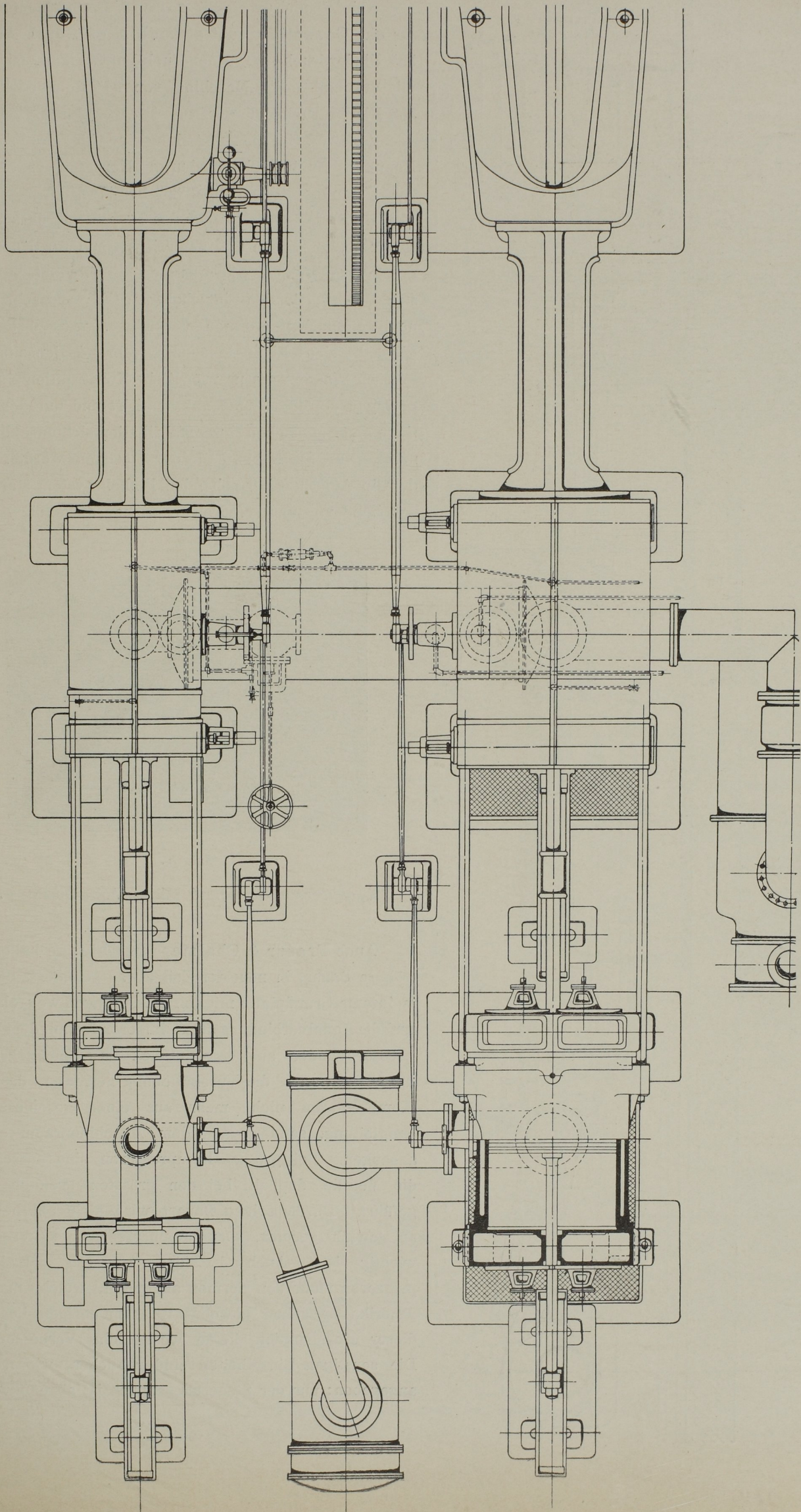
Abb. 68. Grundriss der Maschine. Massst. 1 : 48.
