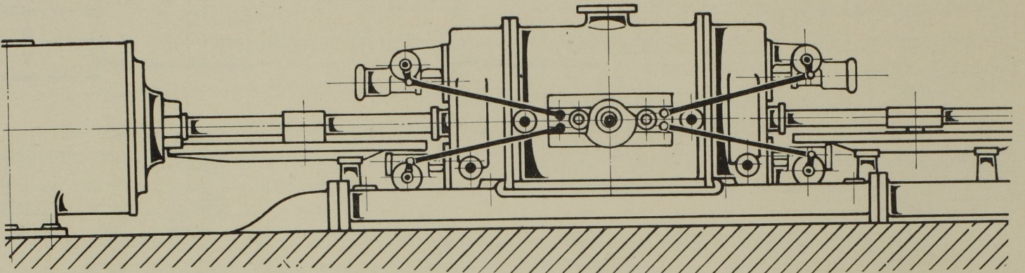
Abb. 4. Kompressorsteuerung. Masst. 1:50.
