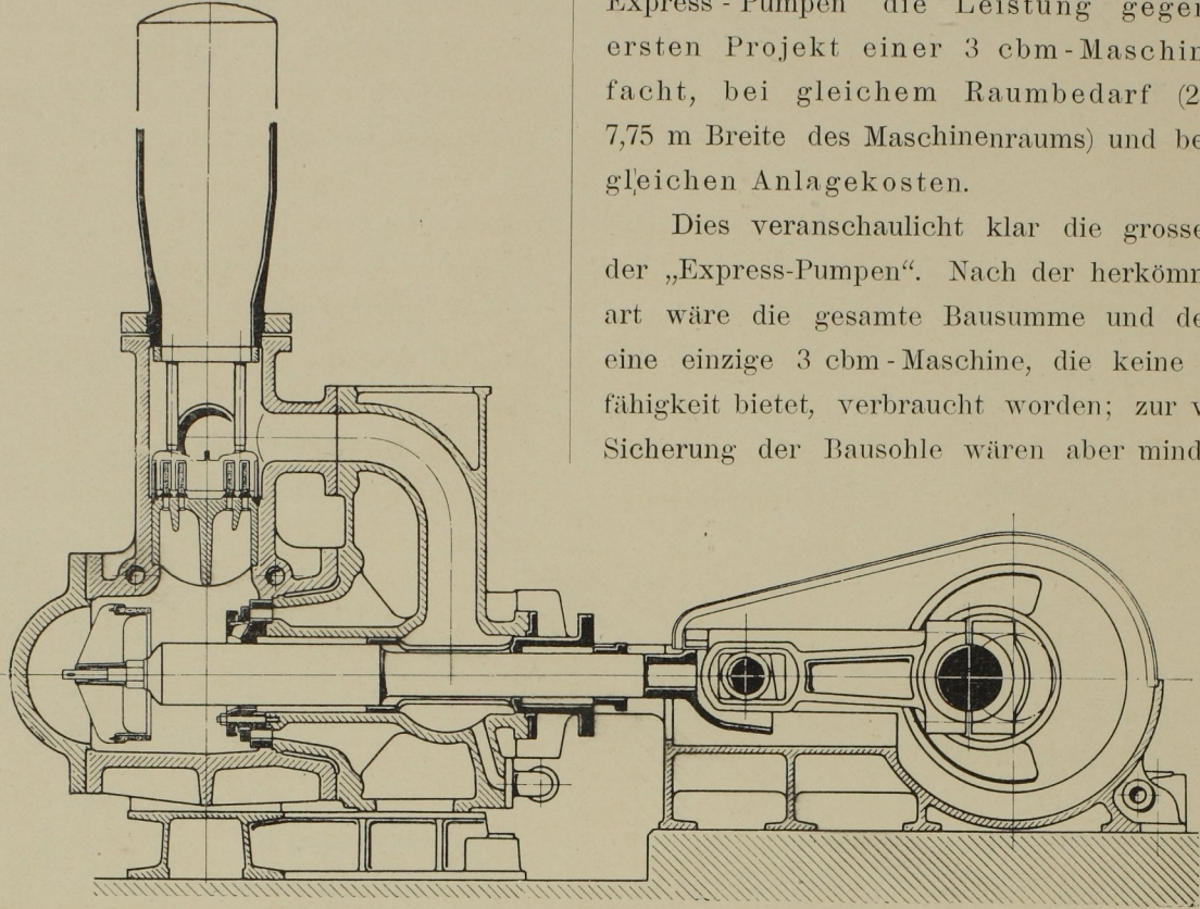
Abb. 19. Längsschnitt der Pumpe. Massst. 1 : 15.
