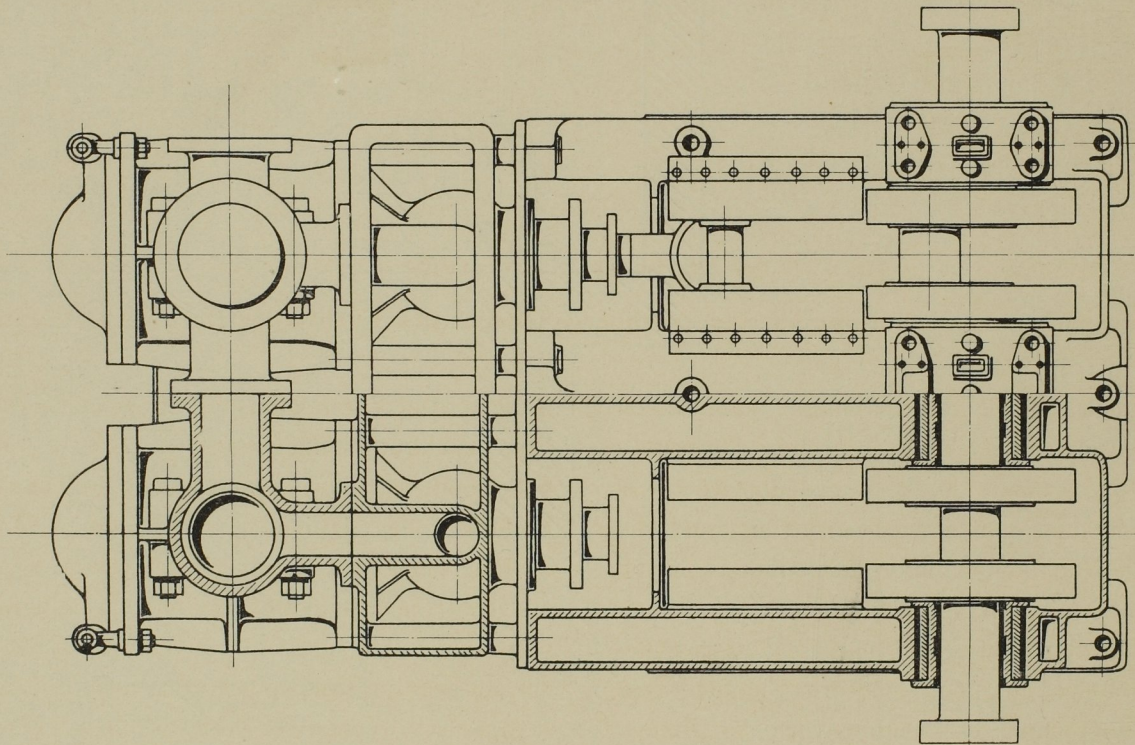
Abb. 20. Grundriss der Pumpe. Massst. 1 : 15.
