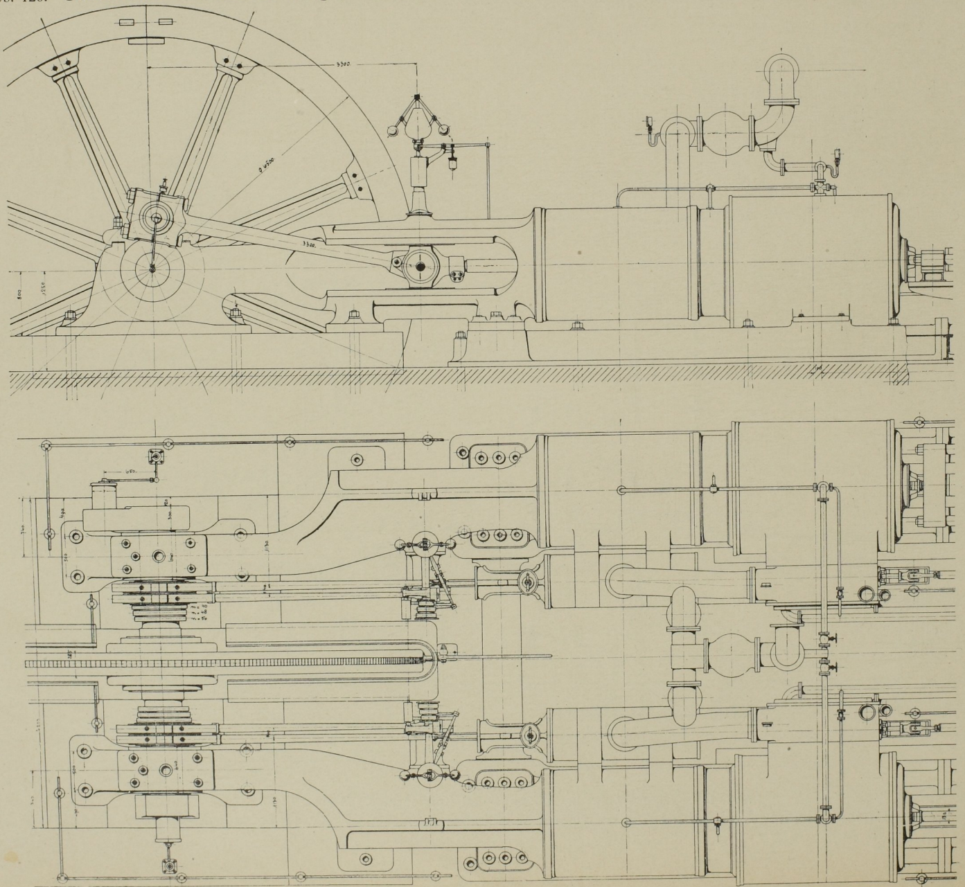
Abb. 121. Unterirdische Zwilling-Tandem-Wasserhaltungsmaschine. Dampfmaschine. Massst. 1:60.
