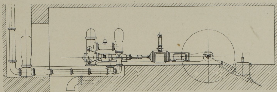
Abb. 108. Wasserhaltung Max-Grube. Masst. 1:200.
